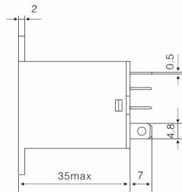
HHC68A(JQX-13F-4Z,LY4)
