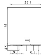
HHC68A-1Z(JQX-13F-1Z/LY1)
