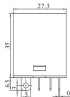
HHC68A-4Z(JQX-13F-4Z/LY4)
