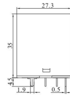
HHC68A-2Z(JQX-13F-2Z/LY2)
