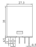
HHC68A(JQX-13F-4Z,LY4)
